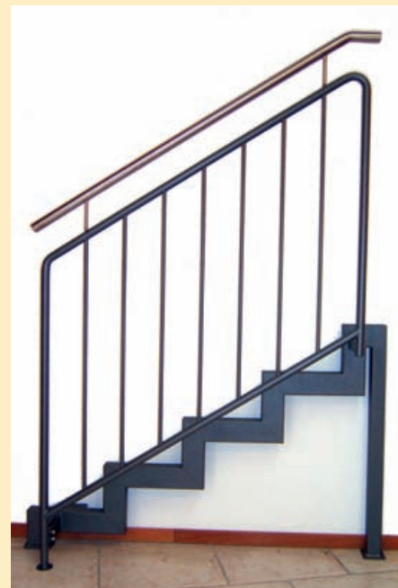
6: Rundrohrgeländer, Obergurt und Untergurt aus Rundrohr 32 mm, senkrechte Füllstäbe 12 mm, Rundrohrpfosten, aufgesetzter Rundrohrhandlauf
