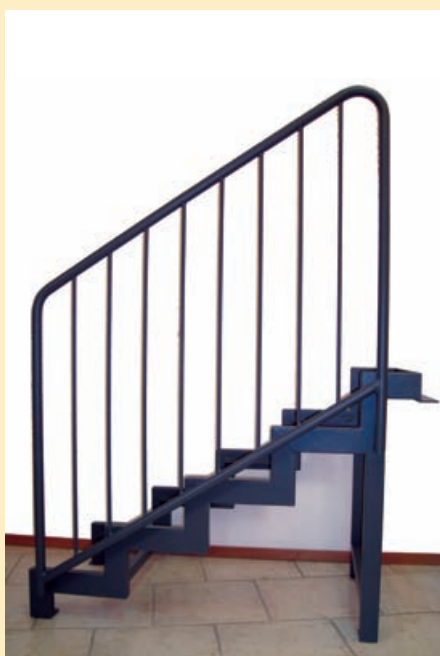
5: Rundrohrgeländer, Obergurt und Untergurt aus Rundrohr 32 mm, senkrechte Füllstäbe 12 mm Durchmesser, Pfosten aus Rundrohr
